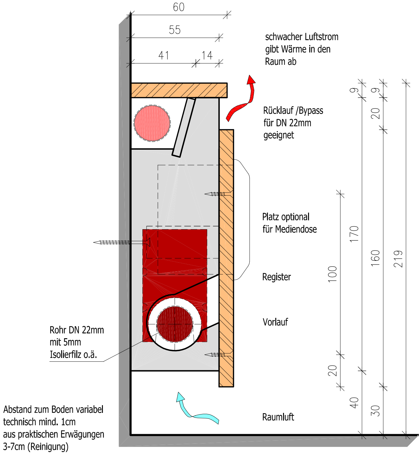
Seitenansicht mit Verkleidung
